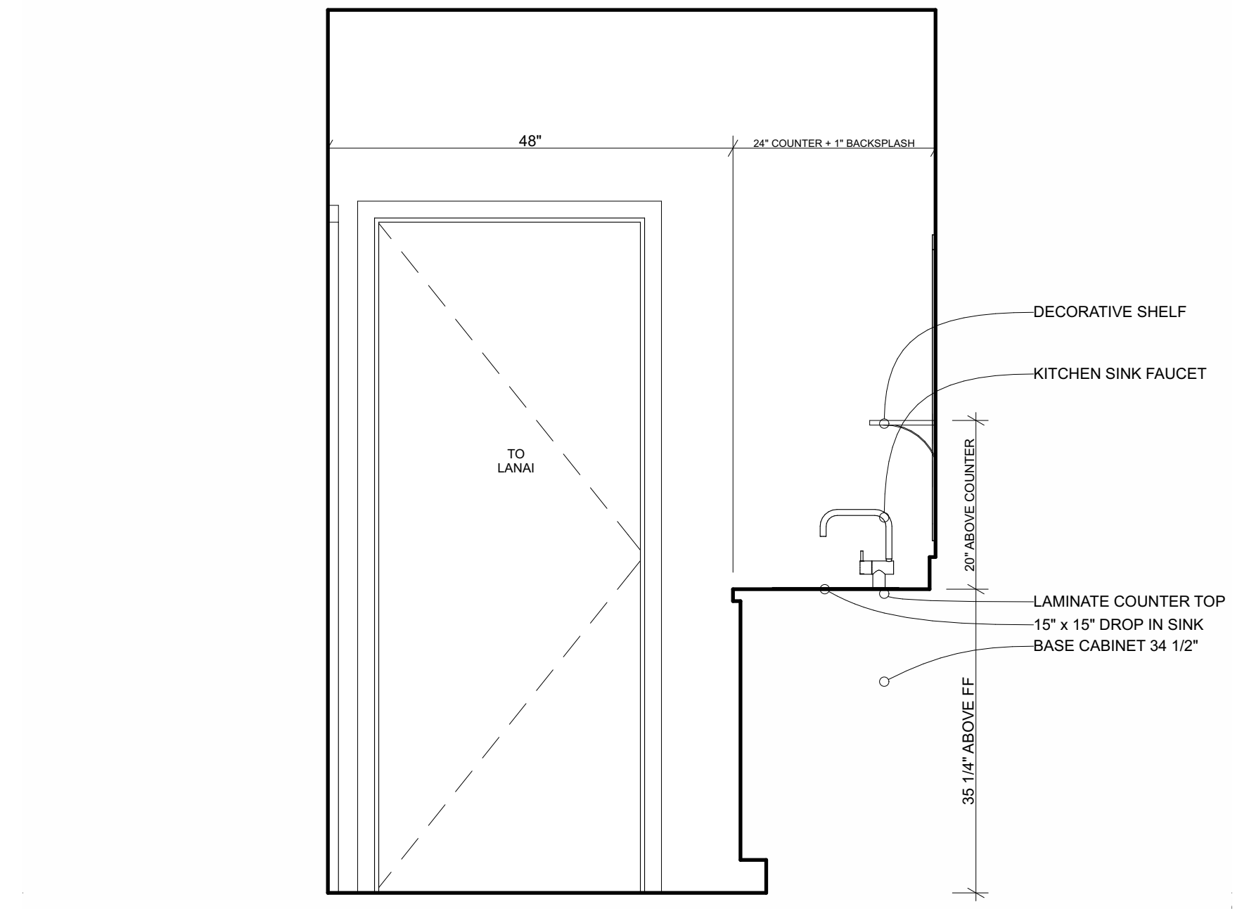
1 A202 LANAI DOOR WALL SCALE: 3/4" = 1'-0"
