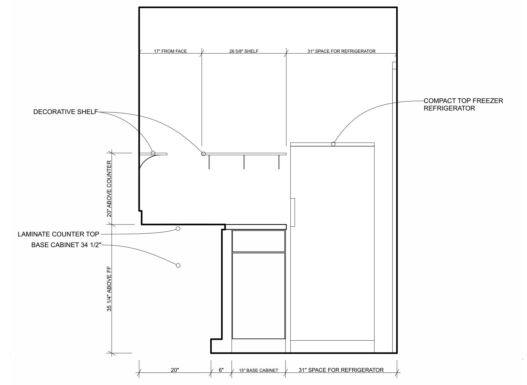
4 A202 REFRIGERATOR WALL SCALE: 3/4" = 1'-0"
